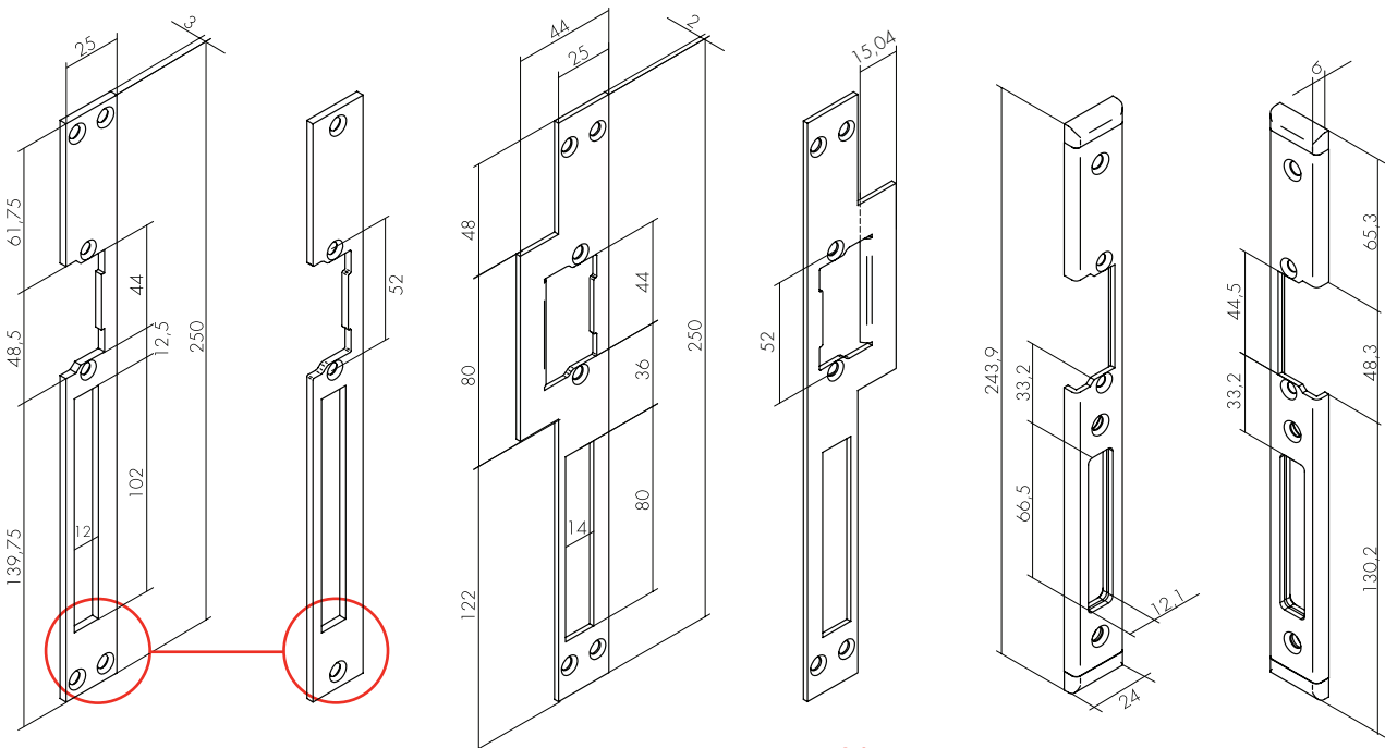
Reversible 05 GREY BROWN Reversible C65 SST 3mm DIN Right 20 SST 2mm DIN left 21 SST 2mm DIN Right 22 SST 3mm DIN Left 23 SST 3mm 65 SST 3mm
