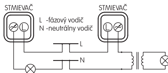
Zapojenie stmievateľa do elektrického obvodu
